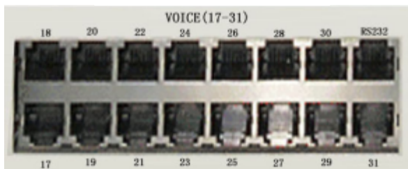
语音接口 17~30
